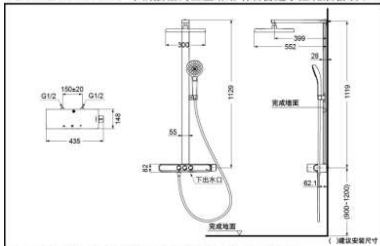
TBW12480CX1X 单柄按钮式恒温淋浴明装普通水压花洒套装 (MY5系列)
