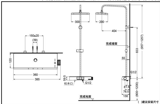
TBW12400C 单柄按钮式恒温淋浴(浴缸)明装普通水压水嘴(带固定花洒与置物台)(L系列)
