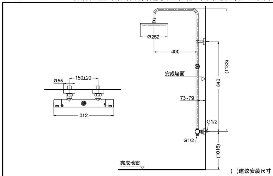
TBW11470C 双柄恒温淋浴明装普通水压水嘴(带固定花洒) (L系列)
