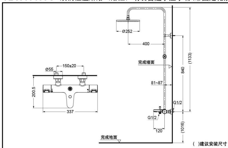
TBW11460C 双柄恒温淋浴（浴缸）明装普通水压水嘴（带固定花洒）（L系列）
