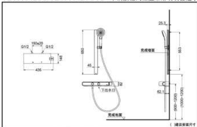
TBW10420C/TBW10420CVD 单柄按钮式恒温淋浴明装普通水压花洒套装 (MY5系列)
