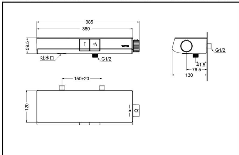
TBV10400C 单柄按钮式恒温淋浴（浴缸）明装普通水压水嘴（带置物台）
