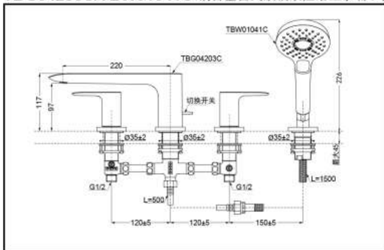
TBG04203C/TBW01041C 铜合金台式双柄双控浴缸水嘴(4孔)(GA系列)
