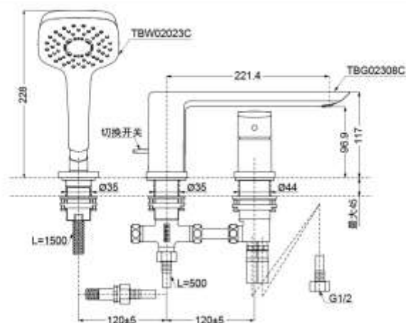
TBG02308C/TBW02023C 铜合金台式单柄双控浴缸水嘴(3孔)(GR系列)
