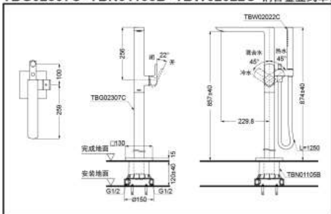
TBG02307C+TBN01105B+TBW02022C 铜合金立式单柄双控浴缸水嘴 (GR系列)
