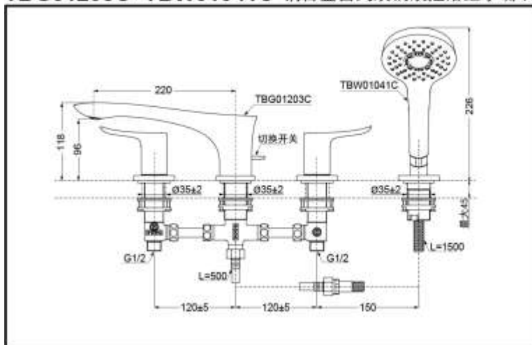
TBG01203C+TBW01041C 铜合金台式双柄双控浴缸水嘴(4孔)(GO系列)
