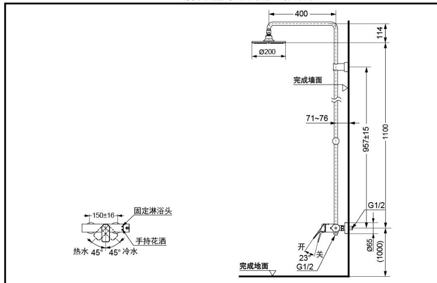
DM919CAR/DM919CA1 铜合金单柄双控淋浴柱
