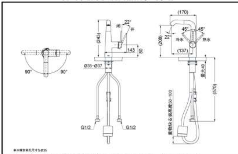
TLS073J0C 台式单柄双控洗面器抽取式水嘴
