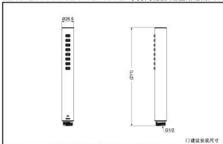
TBW02016C3/TBW02016C2 手持式花洒(浴室淋浴用)(G系列)
