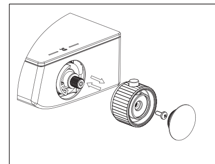
如图为安装把手，锁好螺钉，盖上把手盖完成温度设定
