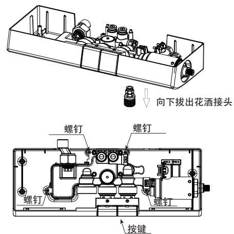
4 将花洒接头拔出，并松脱外壳螺钉，取下本体外壳
