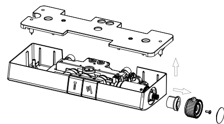
2 用十字螺丝刀拆下盖板及旋钮
