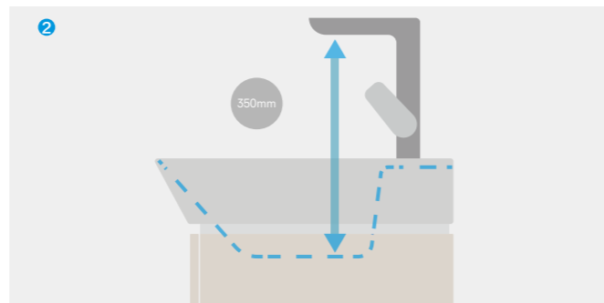
搭配抽拉水嘴，总深度达到 350mm，方便洗头。
